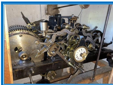
Horloge mécanique MAYET à carillon Westminster
