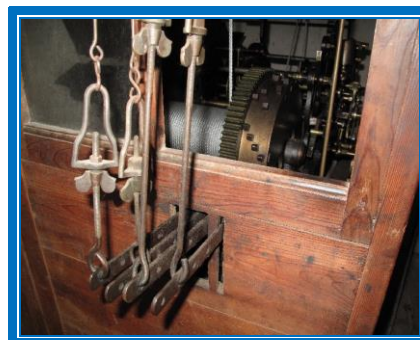
Horloge mécanique MAYET à carillon Westminster
