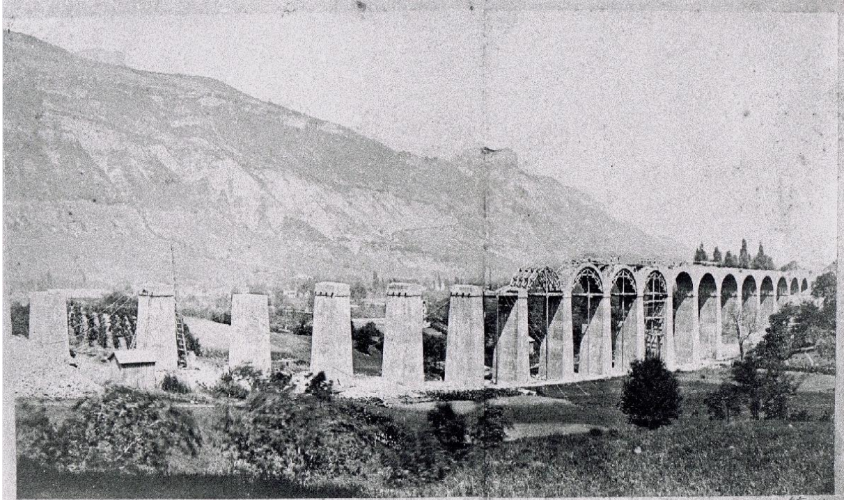
Viaduc du Crozet à VIF (Isère) DU CROZET Ligne Grenoble-Gap
